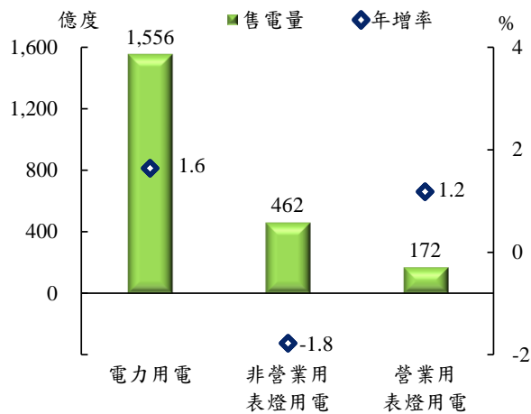
107 年售電量及年增率
